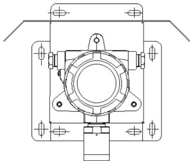
5.3.4 防雨罩管道安装
